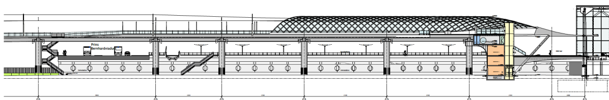
Fig. 2 Longitudinal section.
